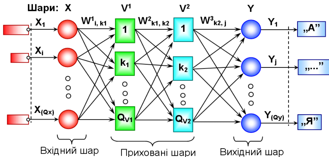
Рисунок 2.4 – Структура багатошарової ШНМ
