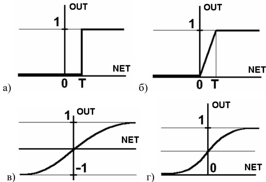
Рисунок 2.3 – Функції активації: а) порогова бінарна функція; б) лінійна обмежена функція; в) гіперболічний тангенс; г) сигмоїдна функція
