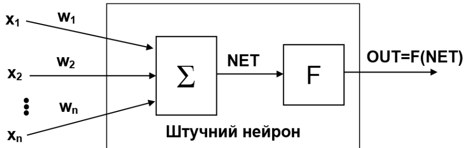
Рисунок 2.2 – Будова штучного нейрону [16]
